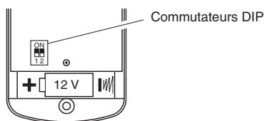
Télécommande dont le panneau arrière est enlevé
