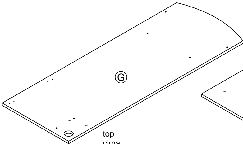
return top cima del retorno dessus du retour 39354026080
