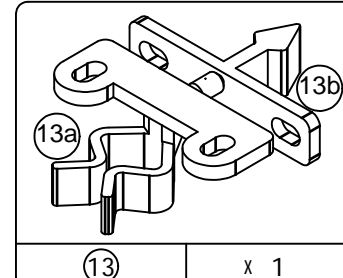
⑬ x 1 #A30030 plastic catch sostenedor plastico loquet en plastique
