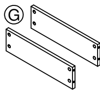
2 aprons 2 delanteros 2 ceintures 31194012070
