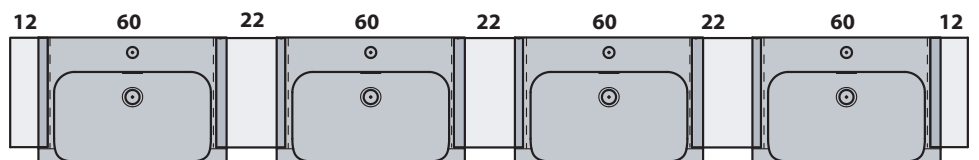
= 314 cm MODULO 4 LAVABI 60 / MODULE 4 WASHBASINS 60
