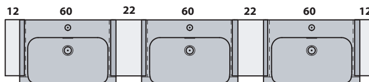
= 236 cm MODULO 3 LAVABI 60 / MODULE 3 WASHBASINS 60
