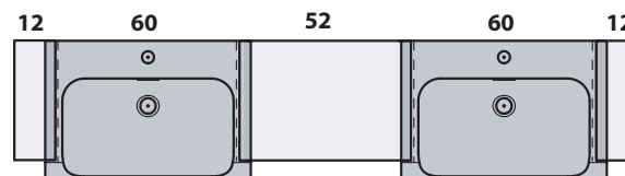
= 188 cm DOPPIA VASCA / DOUBLE SINK
