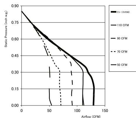
Fan Curve FV-13VKM2
