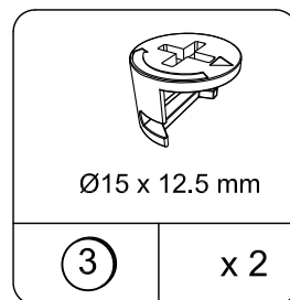
Cam lock Cerradura de la leva TJY0133
