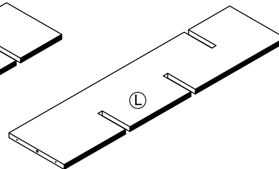
Upper back panel El panel superior de la espalda T1617096120HC
