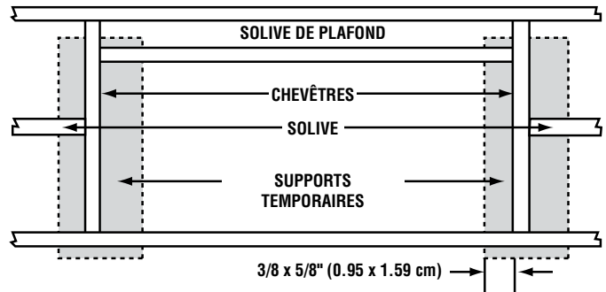
FIGURE 4 – OUVERTURE ENCADRÉE AVEC PANCHETTES DE SUPPORT TEMPORAIRE PRÊTE À RECEVOIR L'ÉCHELLE
